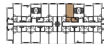
schema podlaží / schematic floor plan
